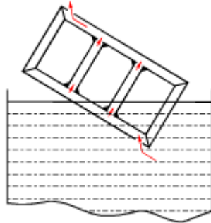
slika 4 – Nevidljivi otvori na cevnoj konstrukciji
